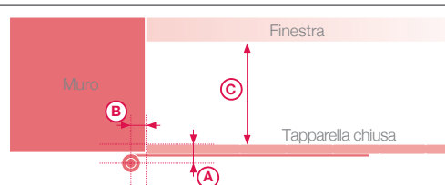
Una tapparella a 2 battenti , peso massimo 30 kg per battente
