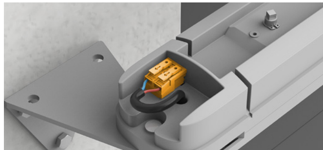
MORSETTIERA DI SERRAGGIO SENZA ATTREZZI
